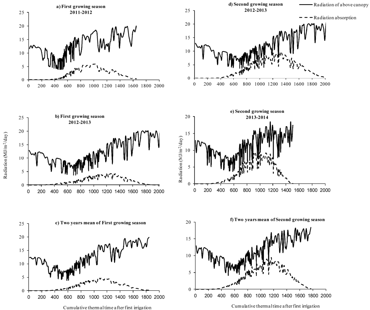
شکل ۳- روند جذب نور زعفران یکساله و دوساله طی فصل رشد
