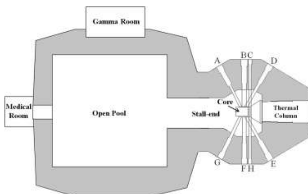
شکل ۱- راکتور تحقیقاتی تهران (Dastjerdi et al., 2016) Figure 1- Tehran Research Reactor (TRR) (Dastjerdi et al., 2016).
