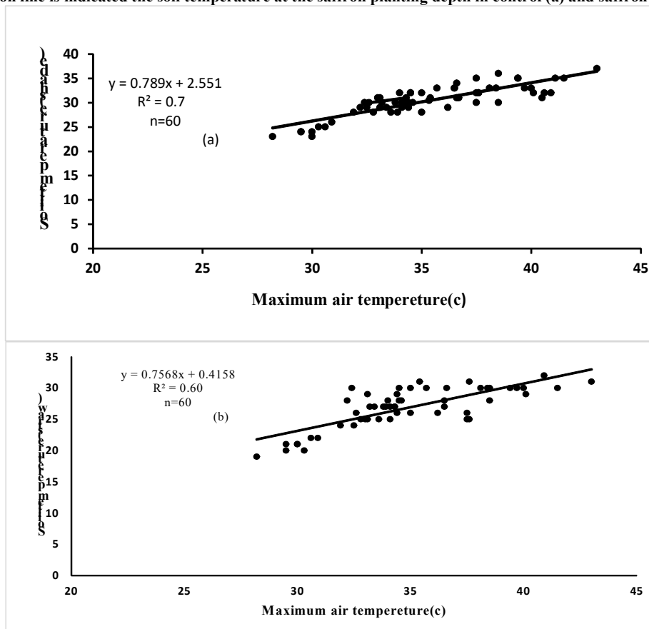
شکل ۴- تغییرات دمای خاک در عمق کاشت بنبه به عنوان تابعی از حداکثر دمای روزانه هوا، شیب خط رگرسیون نشان دهنده دمای خاک در عمق کاشت زعفران برای سایه بان (a) و کلش غلات (b) می‌باشد
