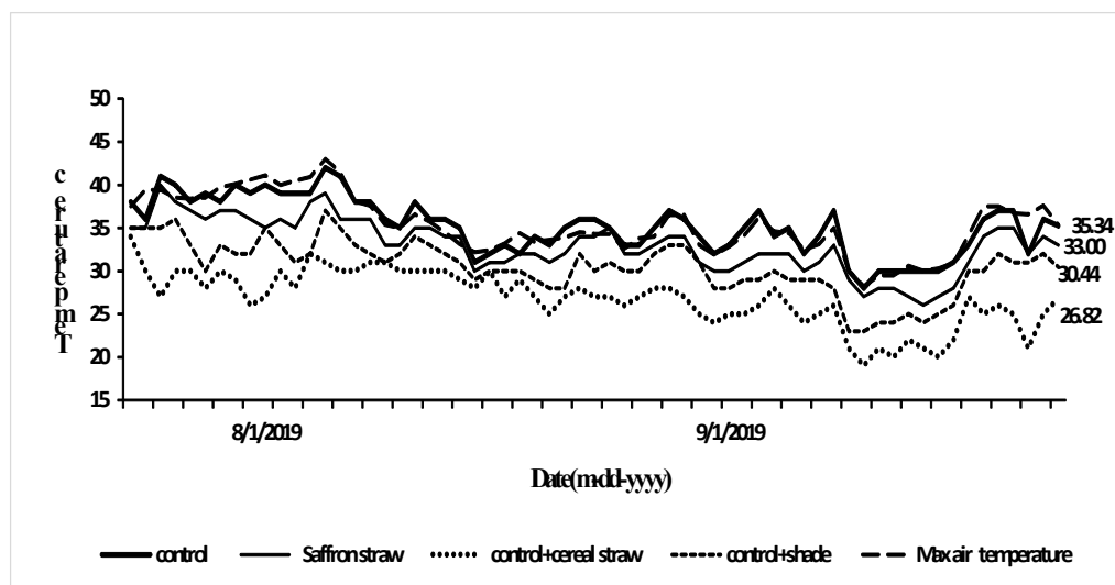
شکل ۲- روند تغییرات حداکثر دمای هوا و دمای خاک در عمق کاشت بونه برای هر یک از سطوح پوشش در طی تابستان (از ابتدای مرداد تا پایان شهریور)
