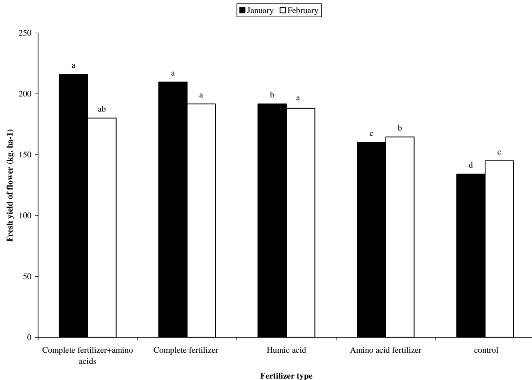
شکل ۲- مقایسه میانگین اثر نوع کود بر عملکرد گل تر زعفران (مقایسه میانگین تیمارها برش دهی در زمان مورد استفاده می باشد) Figure 2- Mean comparison for the effect of fertilizer type on flowers fresh weight of saffron (comparison of means was sliced based on time).
