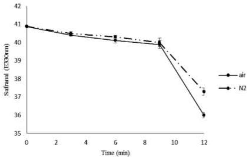
شکل ۷- تأثیر نوع گاز و مدت زمان تابش پلازما بر میزان سافرانال Figure 7- Effect of gas type and exposure of plasma irradiation on safranal.
