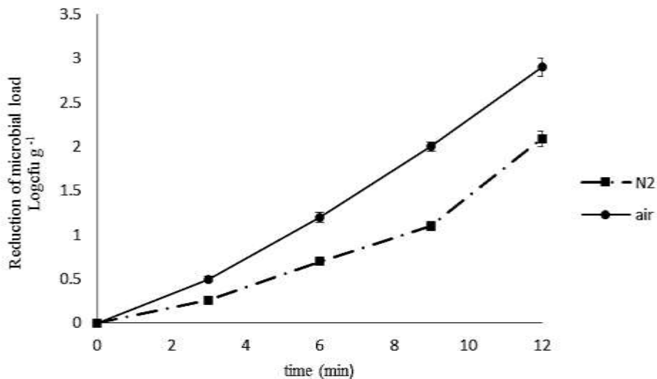
شکل ۲- تأثیر نوع گاز و مدت زمان تابش پلاسمای بر باکتری ائتروکوکوس فکالیس
