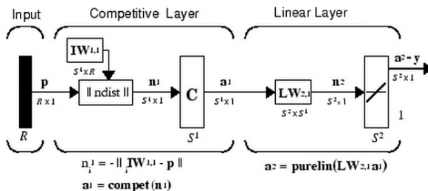
شکل ۲- ساختار شبکه عصبی مصنوعی یک لایه LVQ (Sato & Yamada, 1995) Figure 2- The structure of the LVQ one-layer artificial neural network (Sato & Yamada, 1995).
