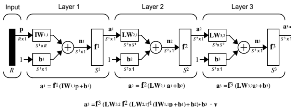
شکل ۱- ساختار شبکه عصبی مصنوعی سه لایه پرسپترون در این مطالعه (Gardner & Dorling, 1998) Figure 1- The structure of the perceptron three-layer artificial neural network in this research (Gardner & Dorling, 1998).
